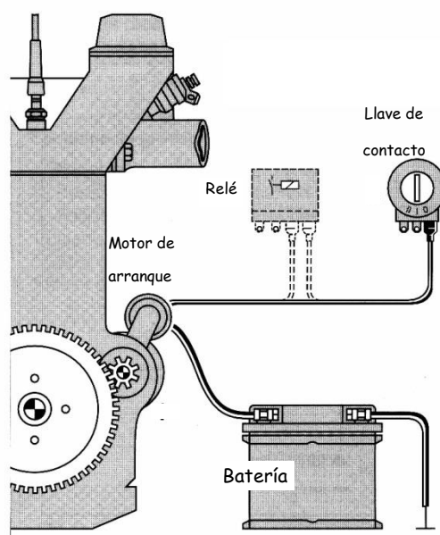
Fig. 12 Situación y conexión del motor de arranque
