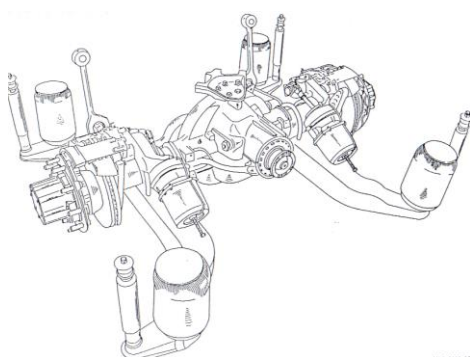
Fig. 19 A mayor carga, mayor cantidad de aire en los fuelles
