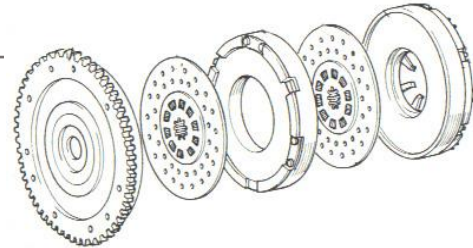
Fig. 5 Despiece de un embrague con dos discos
