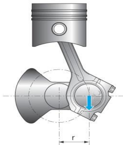
Fig. 22 Esfuerzo de giro
