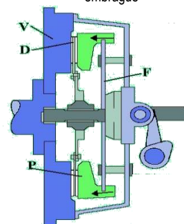
Fig. 7 Embragado
