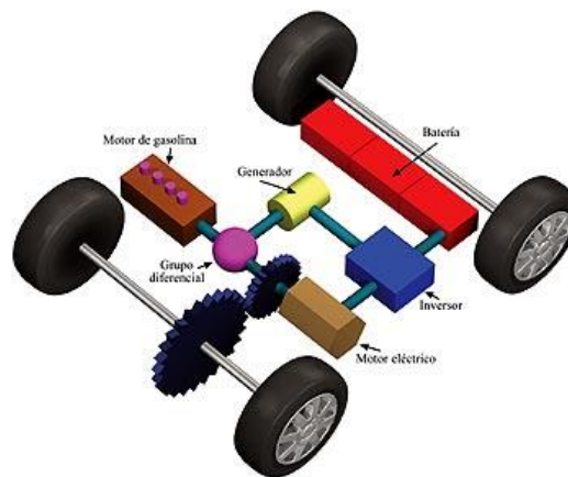
Fig. 25 Situación de los distintos componentes
