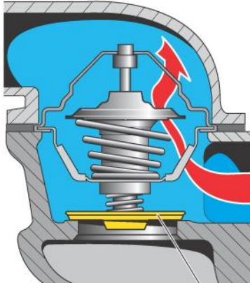
Fig. 19 Termostato abierto
