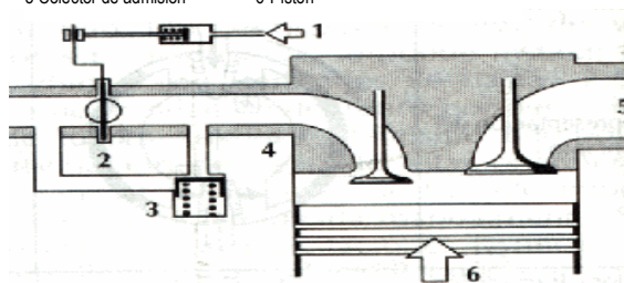
Fig. 10 Freno al escape
