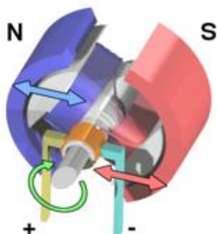
Fig. 28 Campo magnético: la generación del movimiento
