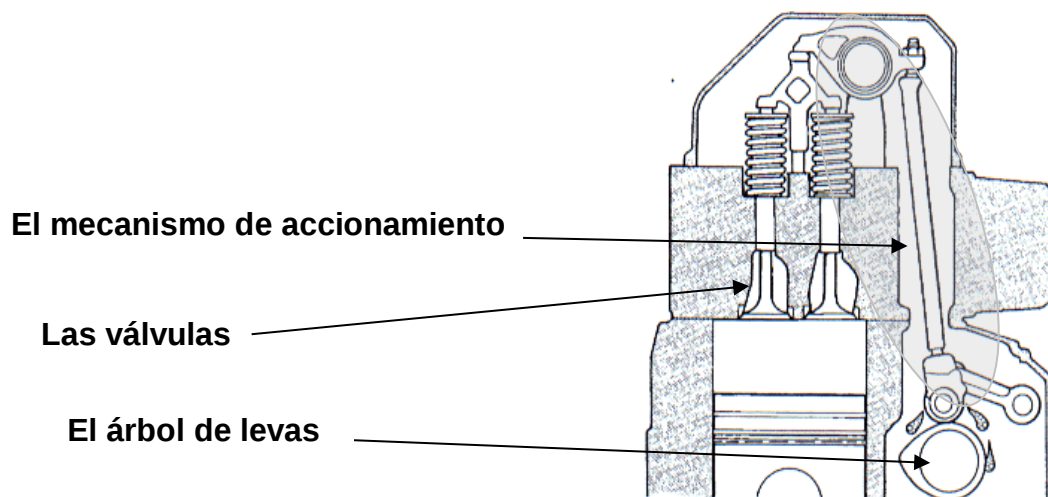
Fig. 10 Sistema de distribución
