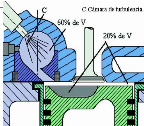
Fig. 3 Inyección indirecta con cámara de turbulencia
