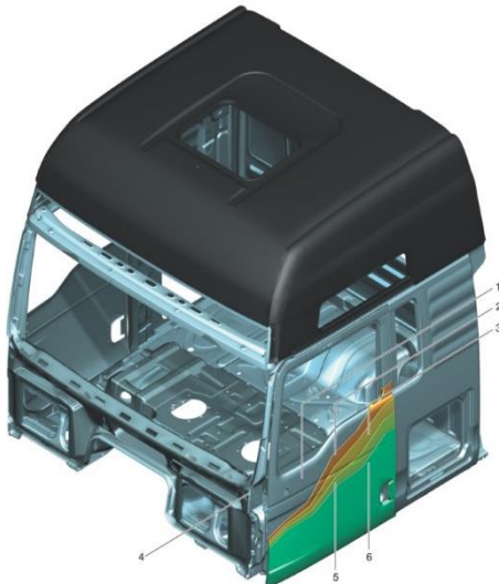
Fig. 5 Cabina: Construcción
