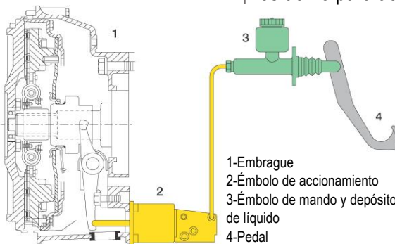
Fig. 9 Accionamiento hidráulico
