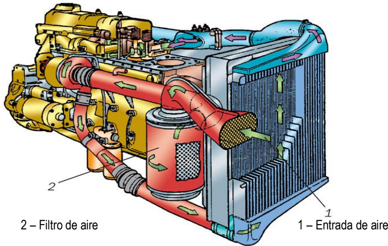
Fig. 1 Sistema de alimentación
