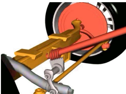
Fig. 4 Conjunto del sistema de dirección
