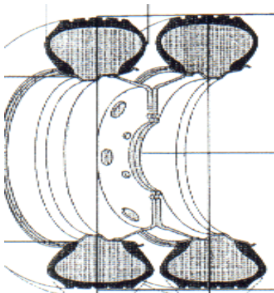
Fig. 14 Montaje gemelo
