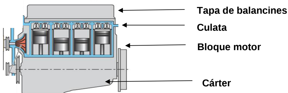
Fig. 2 Conjunto motor
