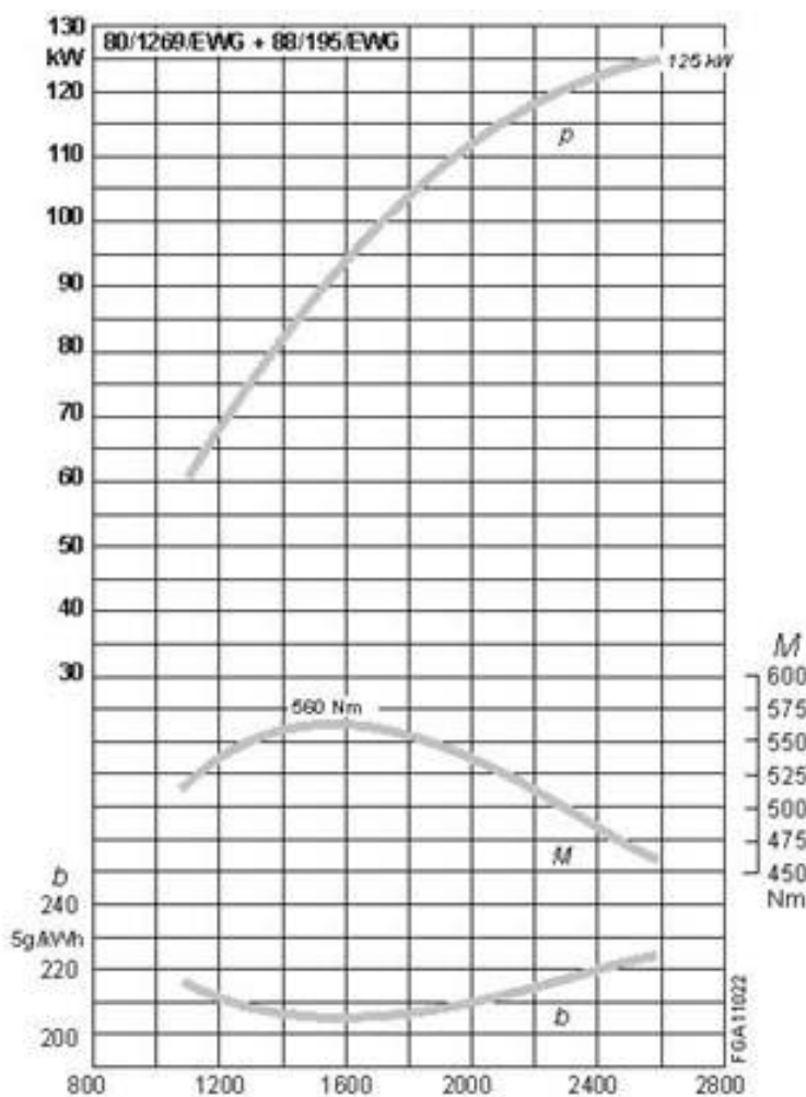
Fig. 23 Curvas de potencia, par y consumo
