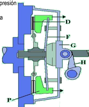
Fig. 8 Desembragado
