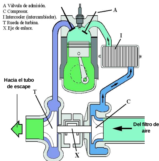
Fig. 12 Recorrido de los gases
