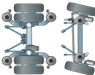
Fig. 3 Distintos montajes de las ruedas
