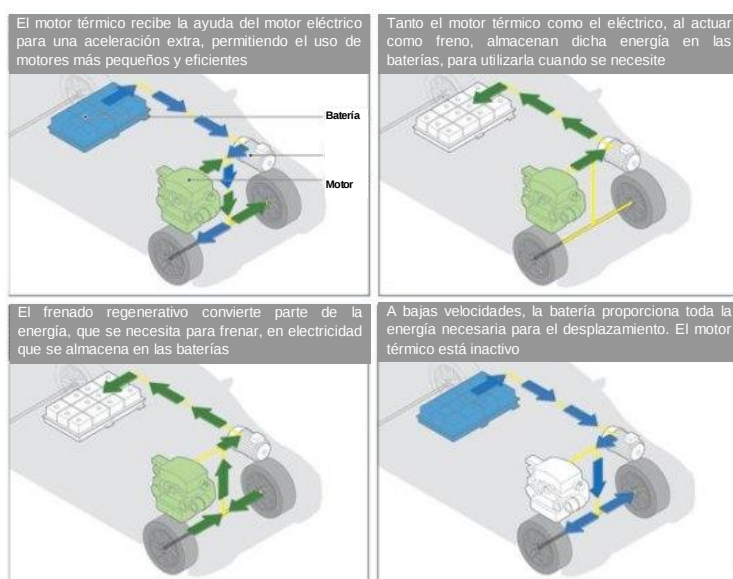
Fig. 26 Flujo de energía
