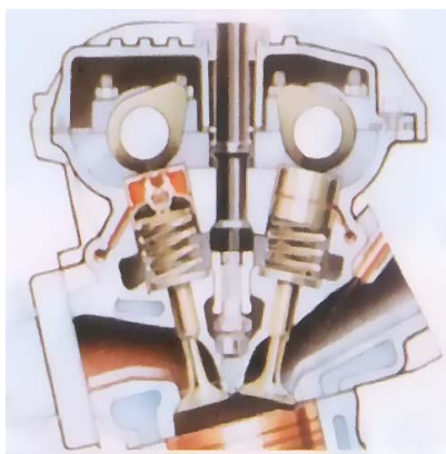
Fig. 11 Válvulas y árbol de levas
