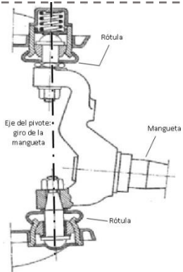
Fig. 5 Conjunto de mangueta-pivote
