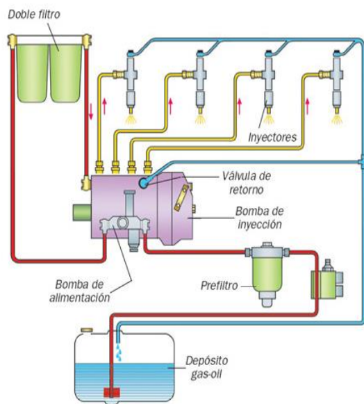
Fig. 15 Sistema mecánico de inyección
