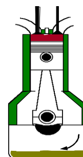
Fig. 19 Combustión
