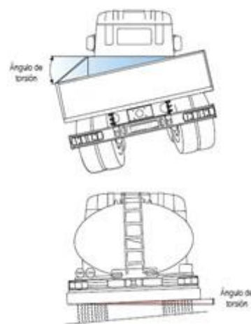
Fig. 17 Movimiento torsional
