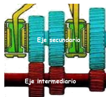
Fig. 14 Constitución de una caja de velocidades
