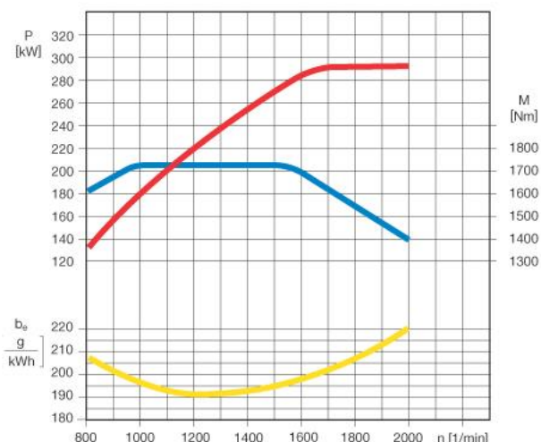
Fig. 24 Curvas características
