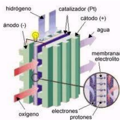
Fig. 30 Generación de electricidad
