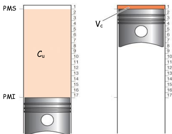
Fig. 21 Relación de compresión
