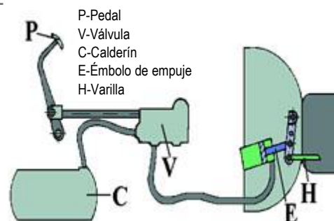
Fig. 10 Accionamiento neumático
